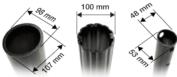
Elliptique 100 mm Aluminium
